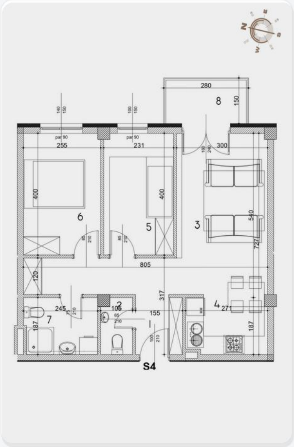
OSNOVA STANA
