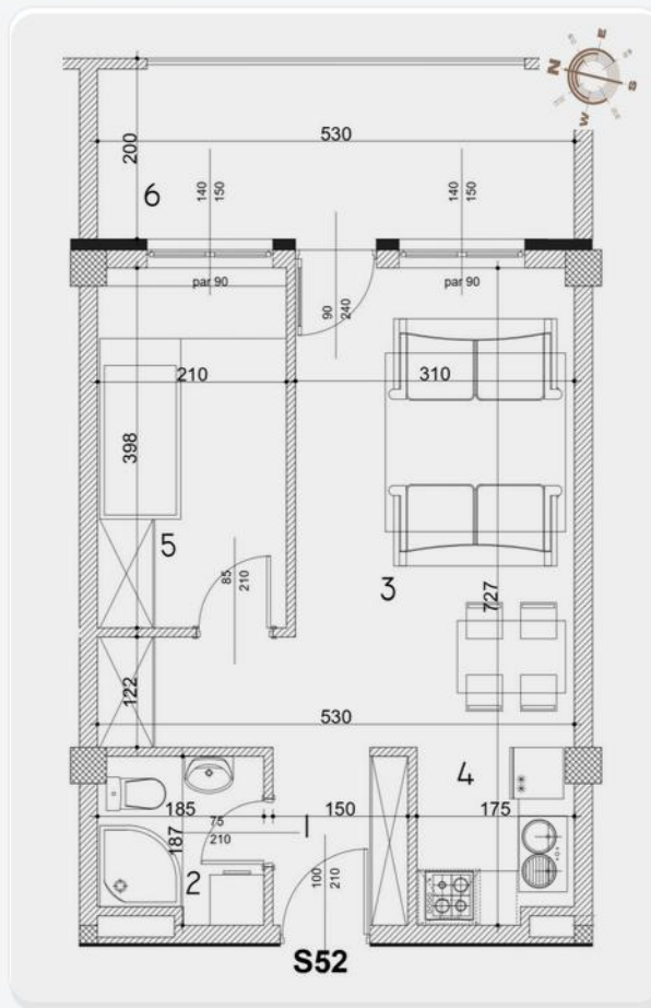
OSNOVA STANA
